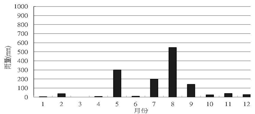
高雄市2015年雨量長條圖
