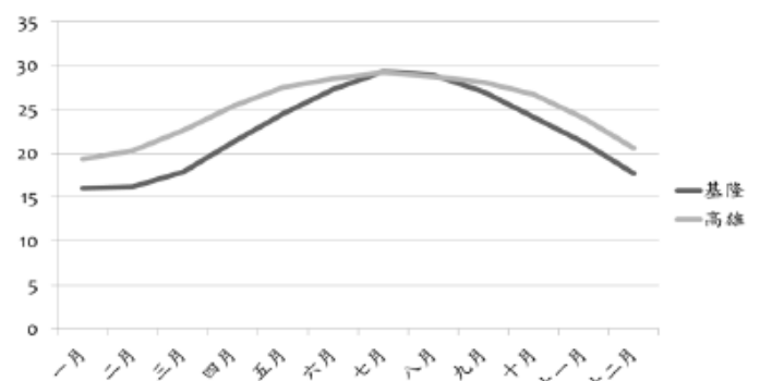
基隆和高雄 (1981-2010) 月均溫比較圖
