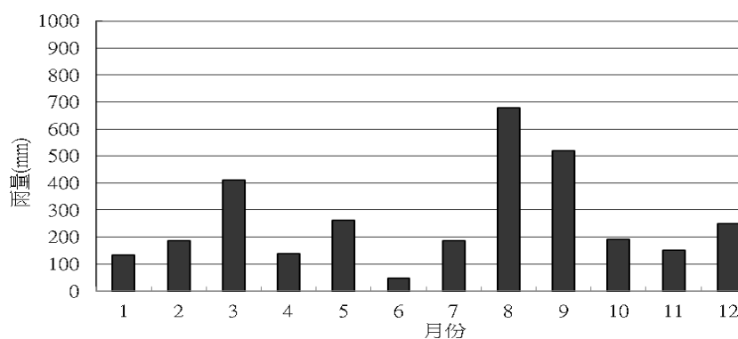
基隆市2015年雨量長條圖
